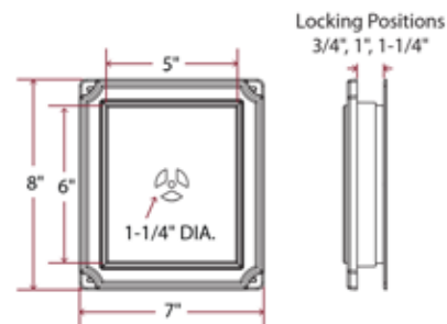
Split Mini
